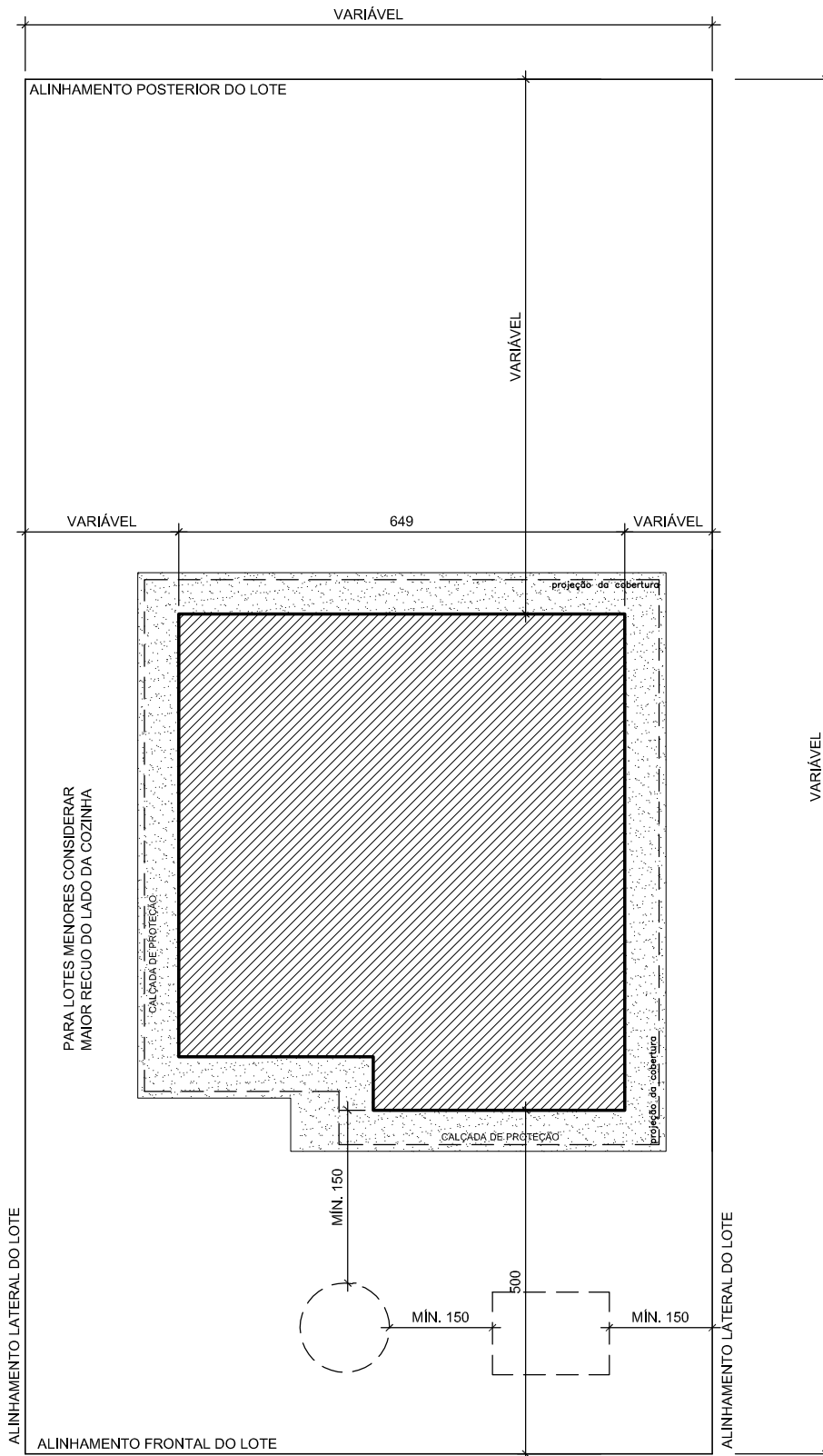
PLANTA MODELO DE IMPLANTAÇÃO ESCALA 1:100
