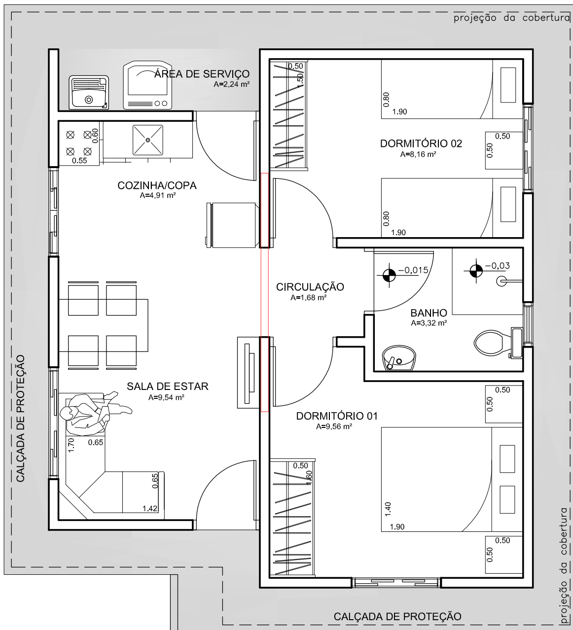
PLANTA TÉRREO - LAYOUT ESCALA 1:50
