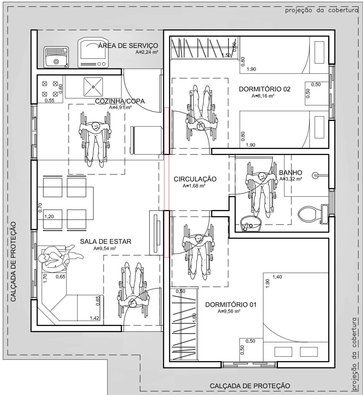
PLANTA TÉRREO - ACESSIBILIDADE ESCALA 1:50
