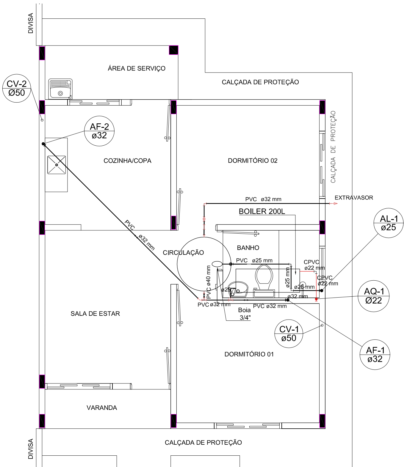
PLANTA COBERTURA - FRIA E ÁGUA QUENTE ESCALA 1:50
