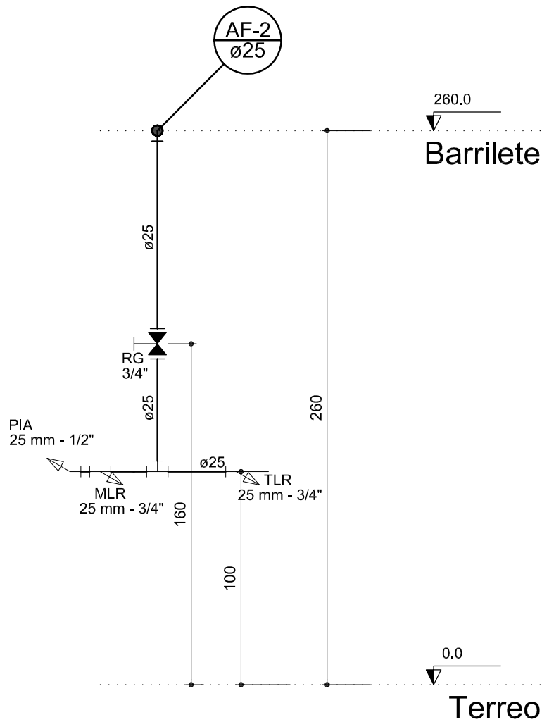
CORTE C3 - ÁREA DE SERVIÇO/COZINHA ESCALA 1:25
