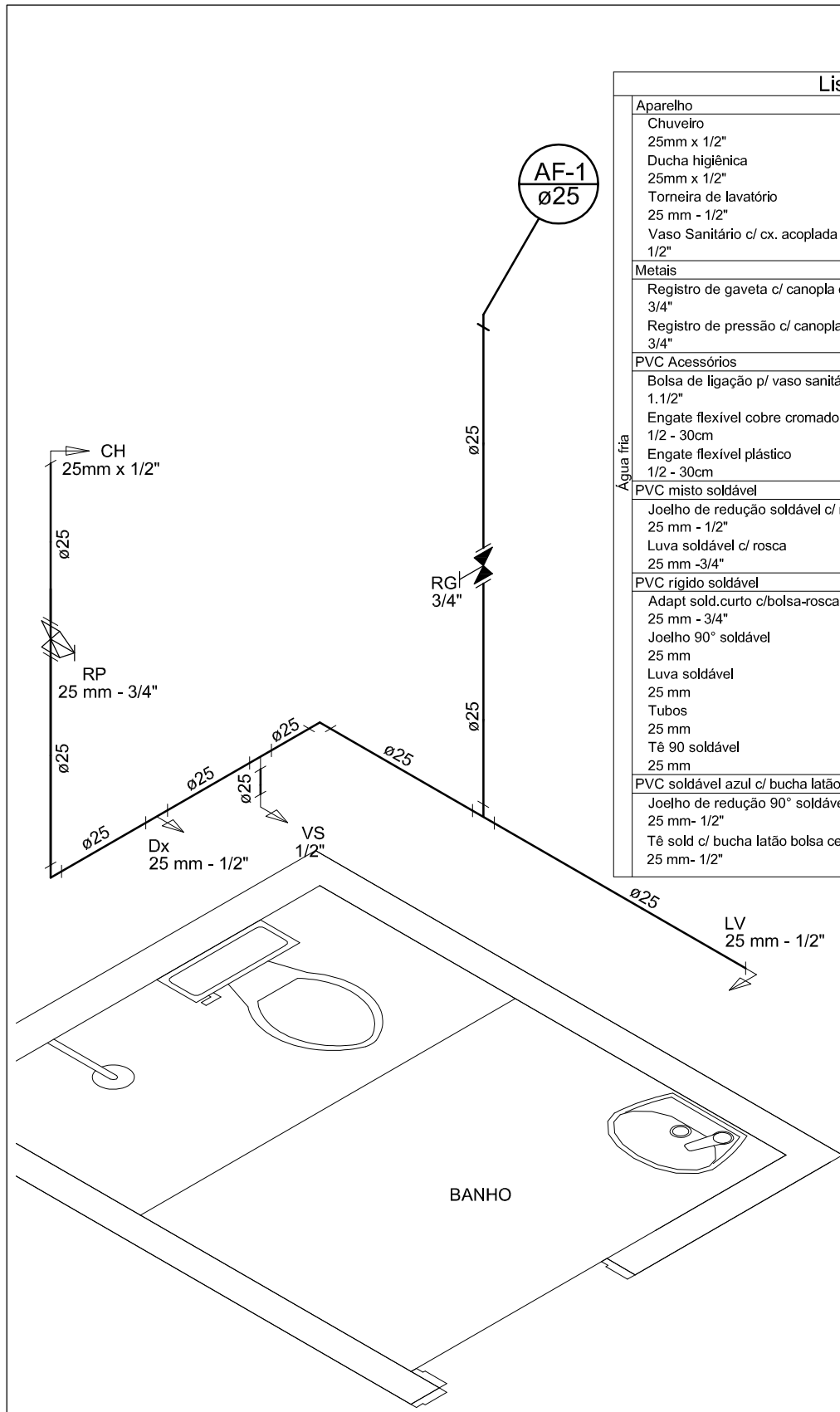
DETALHE ISOMÉTRICO - BANHO ESCALA 1:25
