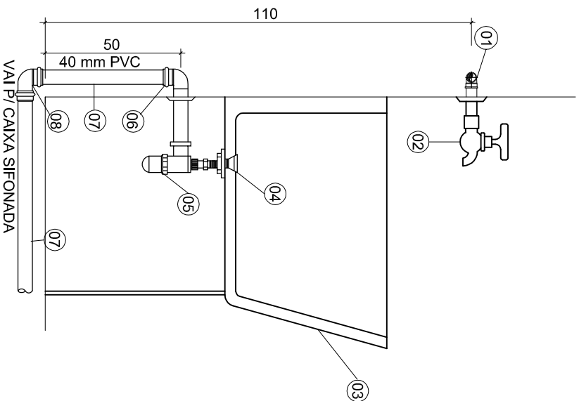
DETALHE MONTAGEM TANQUE SEM ESCALA
