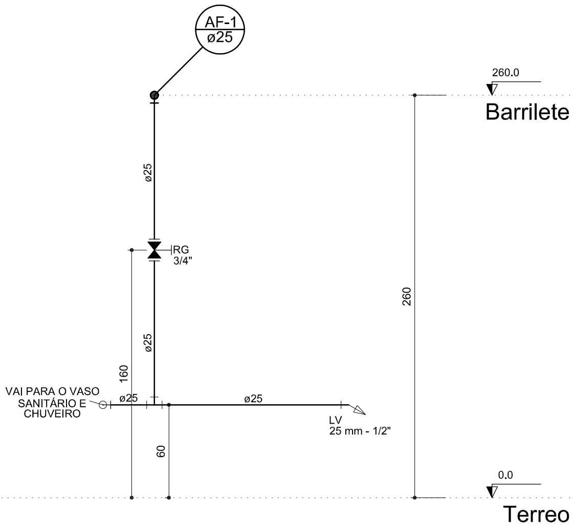
CORTE C1 - BANHO ESCALA 1:25
